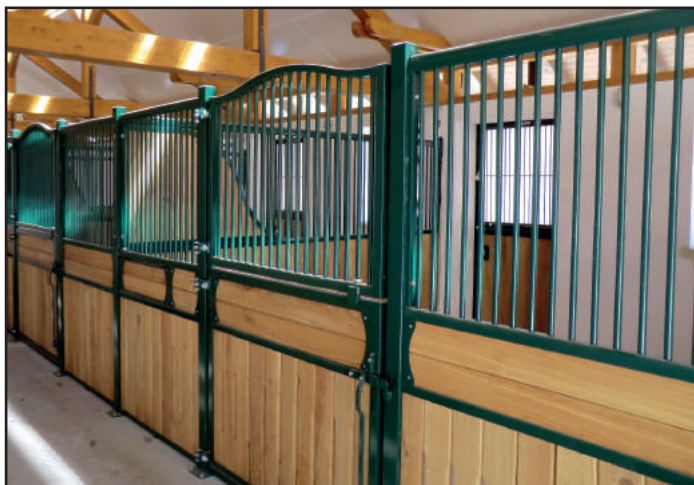
Boxes „Royal“ revêtement plastique vert
