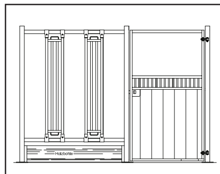
Façade avec cornadis sécurisé et porte pivotante à mi-hauteur
